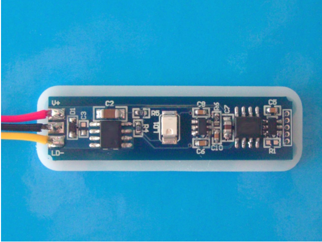
Figura2. Versione con metà guscio frontale in PMMA (vista da dietro) e versione OEM del dimmer (solo scheda).
