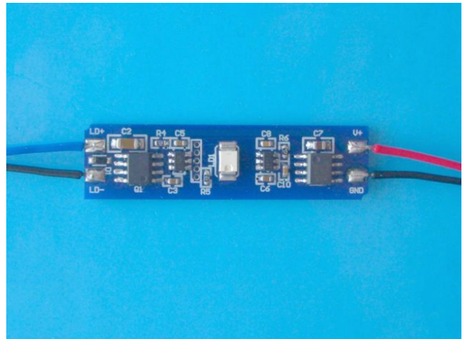
Figura2b. Versione a 4 fili (positivo e negativo di alimentazione su un lato e collegamento anodo e catodo dei led sull'altro lato).
