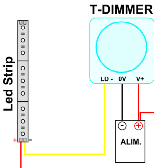
Figura3. Schema di collegamento per la versione a 3 fili.
