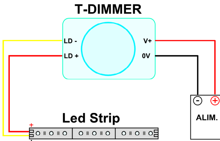
Figura3. Schema di collegamento dei cavi.
