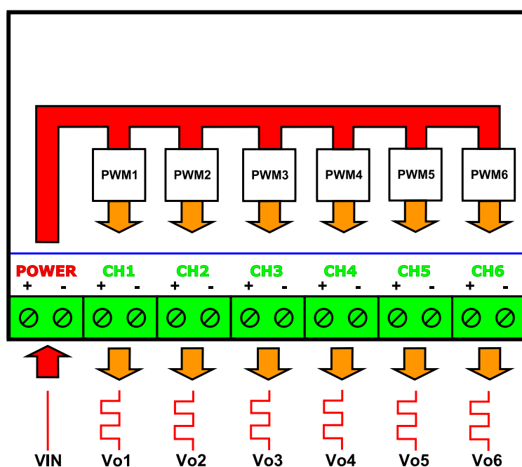
Figura 2. Schema di alimentazione e di uscita.
