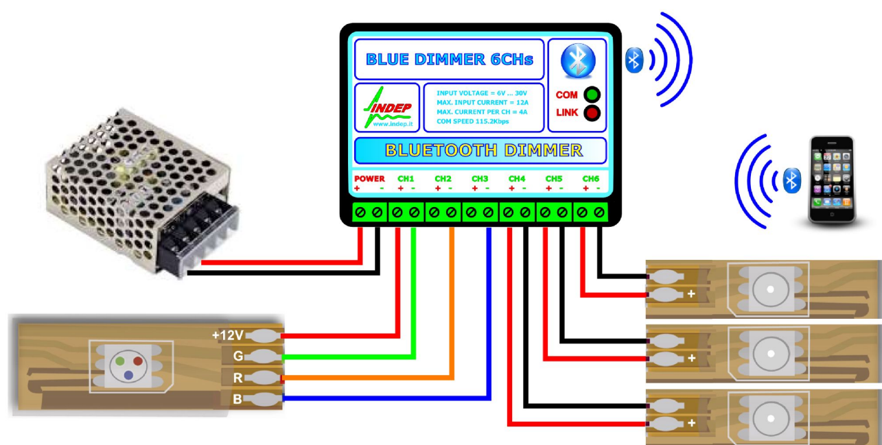
Figura 3. Schema di collegamento di luminarie (strisce led RGB e monocromatiche).
